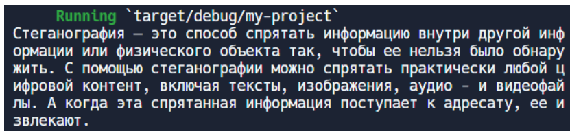
Рис. 4. Декодированная информация
