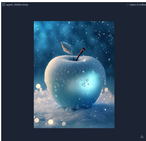
Рис. 3. Выходное изображение
